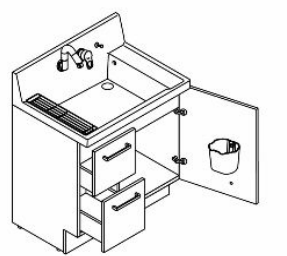
引出タイプ AR3H-755SY/LM2H
